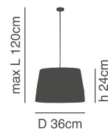
77-3639-50 L-P-1708 1xE27, max 60W, 230V
